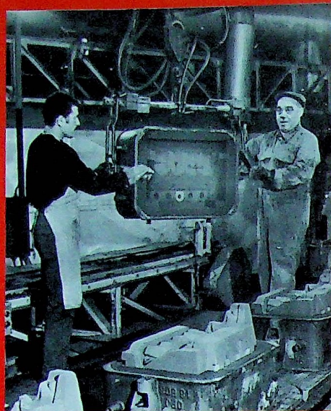
Puis on coiffe le moule de sa partie supérieure, dans laquelle des ouvertures ont été aménagées pour la coulée du métal et l'échappement des gaz.
