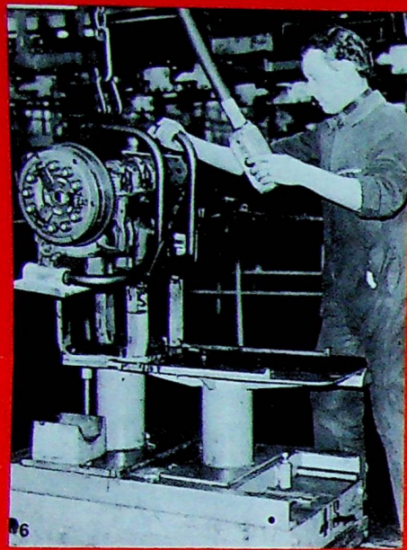
6. Toutes les maintenances sont faites mécaniquement. Voici le départ du carrousel.
