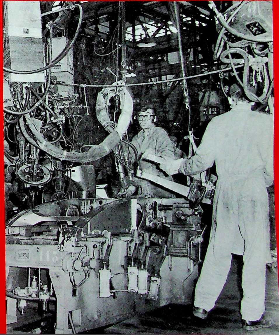
Soudure sur maquette de l'unit-avant du caisson
