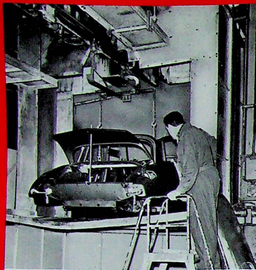
1. L'entrée du tunnel de bondérisation.
