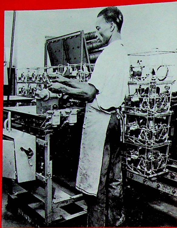
8. Montage des roulements à billes des pivots. Dans chaque panier, l'ensemble des pièces qui constituent le pivot.
