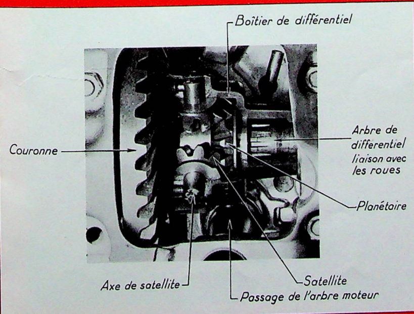
Le différentiel : il permet des vitesses de roues différentes dans les courbes.
