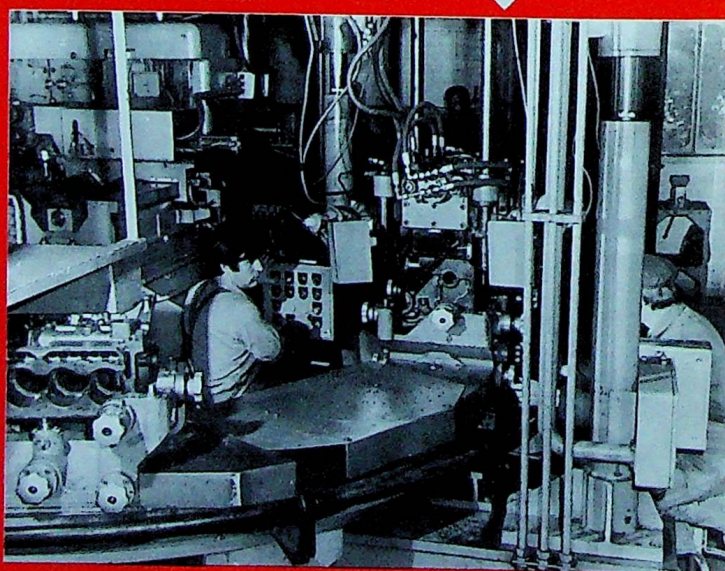
Le carter-moteur est ensuite peint, pour éviter l'oxydation. Il reste à s'assurer que la pièce est usinable. Pour ce faire, elle est présentée sur un montage qui permet de vérifier et de répartir les surépaisseurs d'usinage. Enfin quatre touches sont fraisées sur la pièce : elles serviront de point de départ pour le travail d'usinage.
