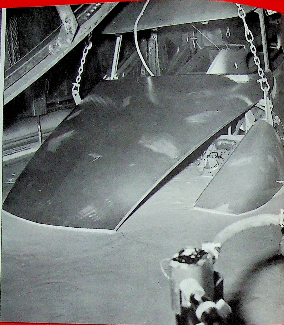
2. La plongée dans la cuve d'électrophorèse (33 mètres de long, 190 000 litres de peinture).
