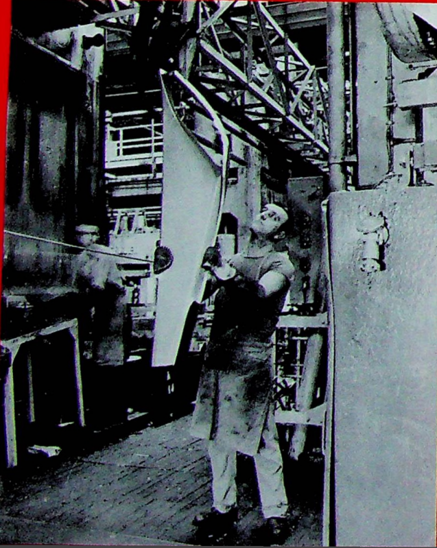
11. Après la mise en forme, la pièce passe sur six presses « simple effet » alignées et travaillant semi-automatiquement pour des opérations de détourages, de percements de « fenêtres » et de trous, de tombages de bords.
