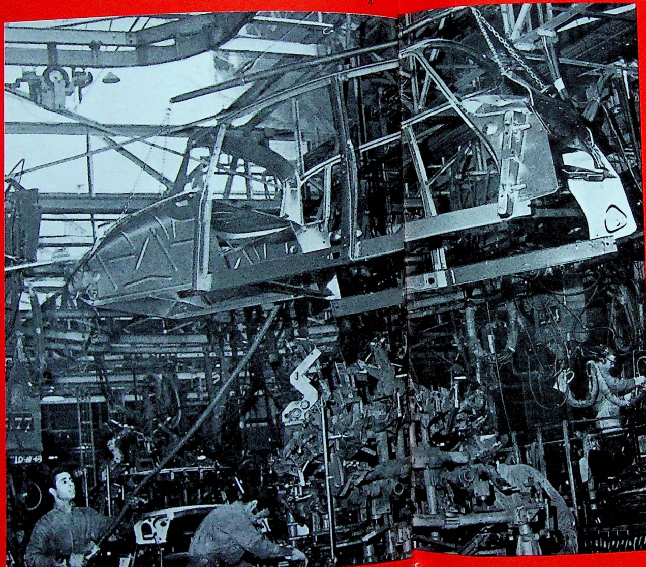
1. Sur ce chariot est déposé l'ensemble du caisson : unit-avant, unit-arrière et plancher. Le chariot, placé sur un carrousel (comportant 17 chariots), progresse automatiquement, et passe sur trois soudeuses multipoints entièrement automatiques.
