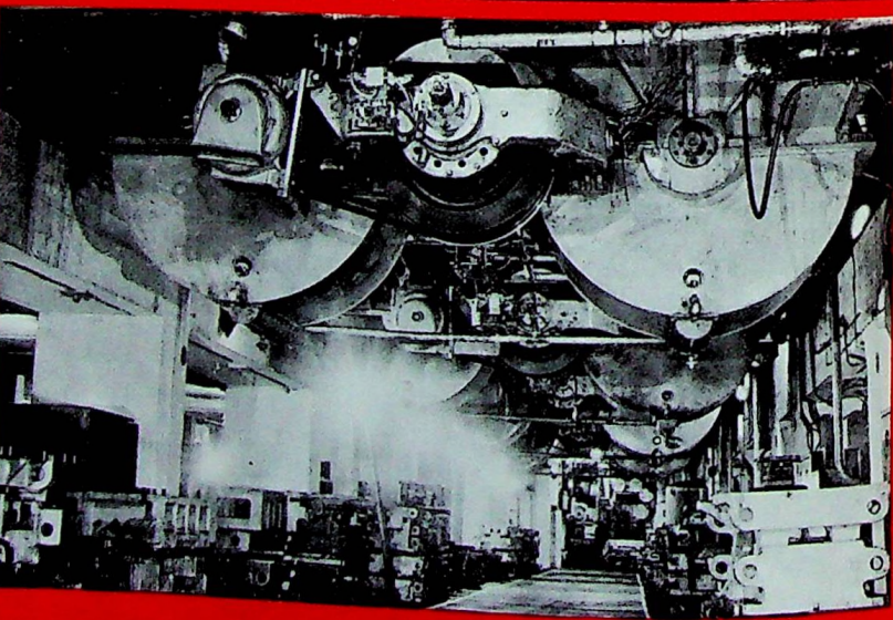
11. Après la mise en forme, la pièce passe sur six presses « simple effet » alignées et travaillant semi-automatiquement pour des opérations de détourages, de percements de « fenêtres » et de trous, de tombages de bords.
