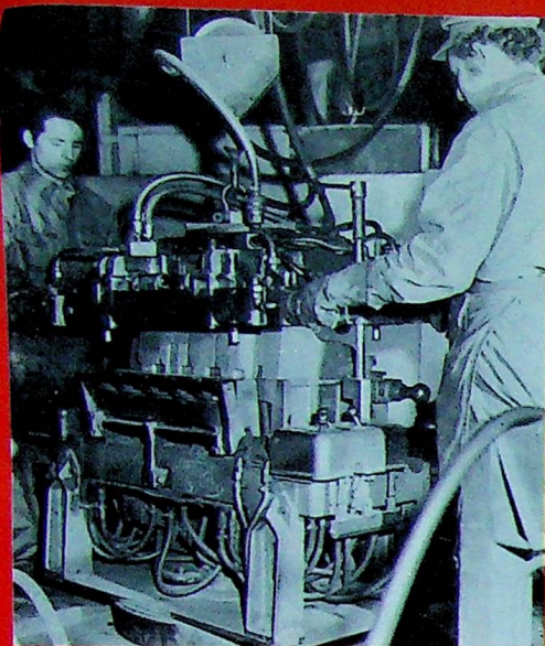
L'ensemble des noyaux est ensuite agrippé et déposé dans la partie inférieure du moule.
