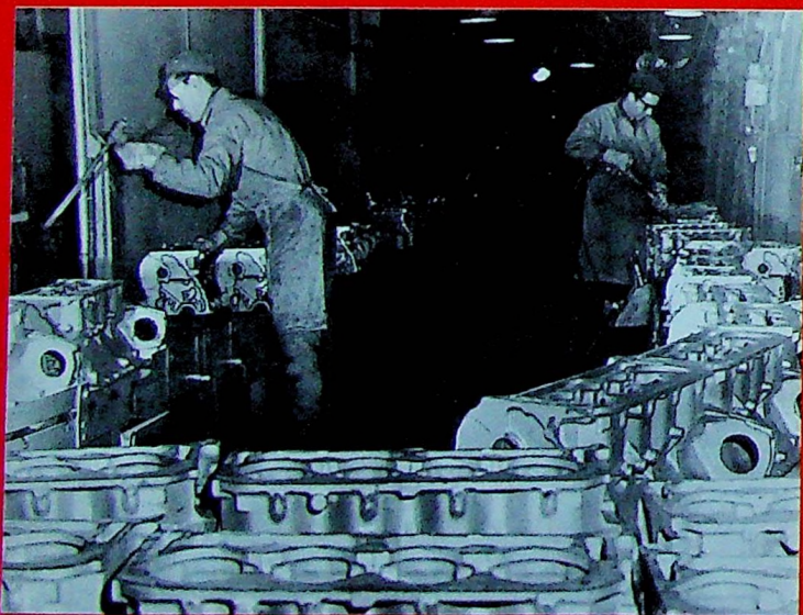
Après un temps de refroidissement, le moule est décoché, le sable en partie récupéré; le carter-moteur apparaît à l'état brut. Il va subir une première opération de décapage par projection de grenailles. Il sera ensuite « ébarbé », opération qui consiste à enlever, à la meule ou au burin, toutes les parties superflues.
