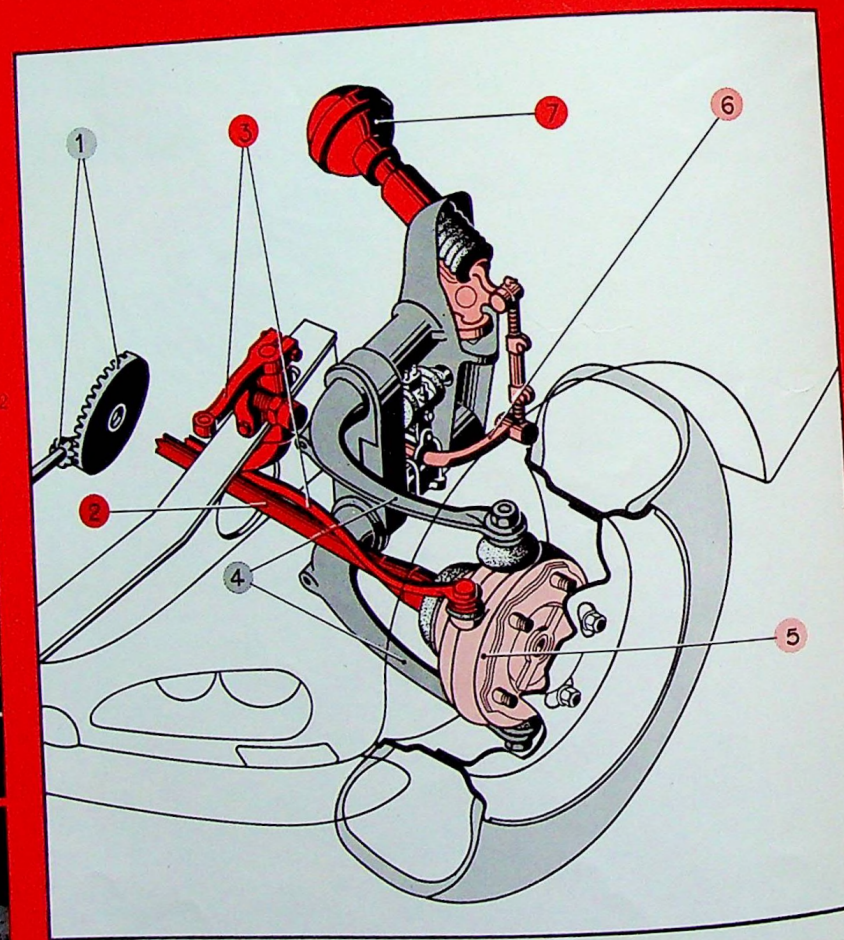
1. L'ensemble couronne-pignon (ou couple conique) : placé en sortie de boîte de vitesses, il transmet la rotation de son arbre secondaire (longitudinal) aux roues (axes perpendiculaires). 2. L'arbre de transmission : il comporte des articulations qui lui permettent de suivre tous les débattements de la roue. 3. La direction : par laquelle le conducteur donne aux roues leur orientation. (Cette partie n'est pas montée à Grenelle : nous l'avons fait figurer pour que le schéma soit complet.) 4. Les demi-essieux avant : rattachent au châssis l'ensemble moyeu-pivot, et permettent les débattements de bas en haut. 5. Ensemble moyeu-pivot : il porte la roue et la relie à l'arbre de transmission (2), les demi-essieux avant (4) et l'organe de direction (3). 6. La barre antiroulis. 7. La sphère assure suspension et amortissement (amortisseur intégré dans la sphère).
