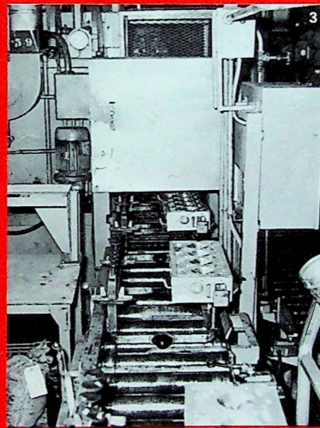
1. Plus d'un kilomètre de convoyeurs aériens domine la chaîne : un signal sonore signale les incidents de parcours, tandis que la panne est localisée sur un tableau lumineux. 2. Les équipes d'entretien interviennent sur-le-champ.
