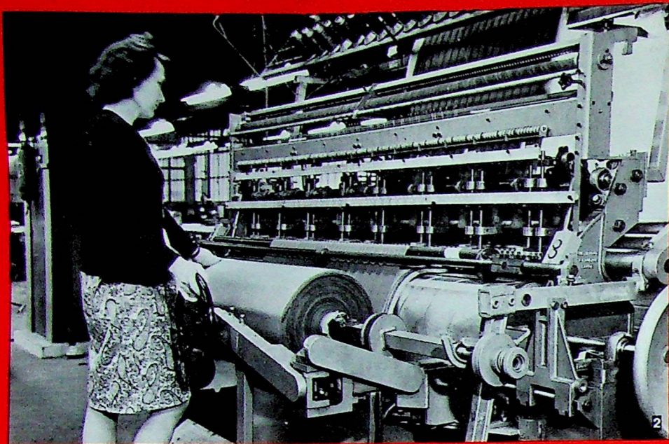
2. Une machine à piquer les côtes (tissu et mousse ensemble) : elle s'arrête lorsqu'un fil casse. Elle est armée de 25 aiguilles et débite 75 mètres à l'heure.
