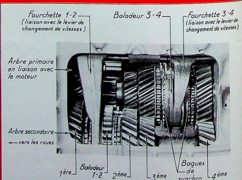
Schema de la boîte de vitesses et transmission de la rotation aux roues.
