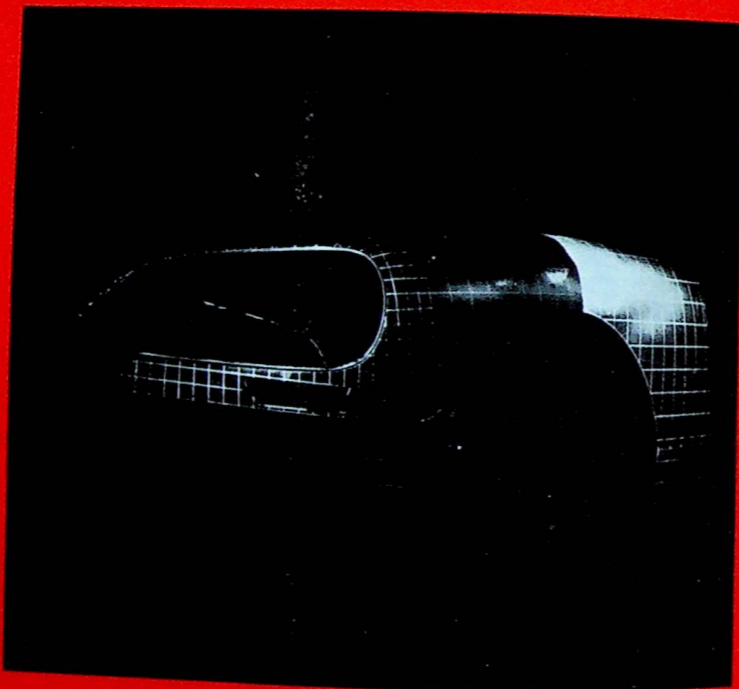
2. Opérations de contrôle sur une aile terminée : sur cette maquette qui positionne l'aile comme si elle était sur la voiture, ce contrôleur prend 41 mesures
